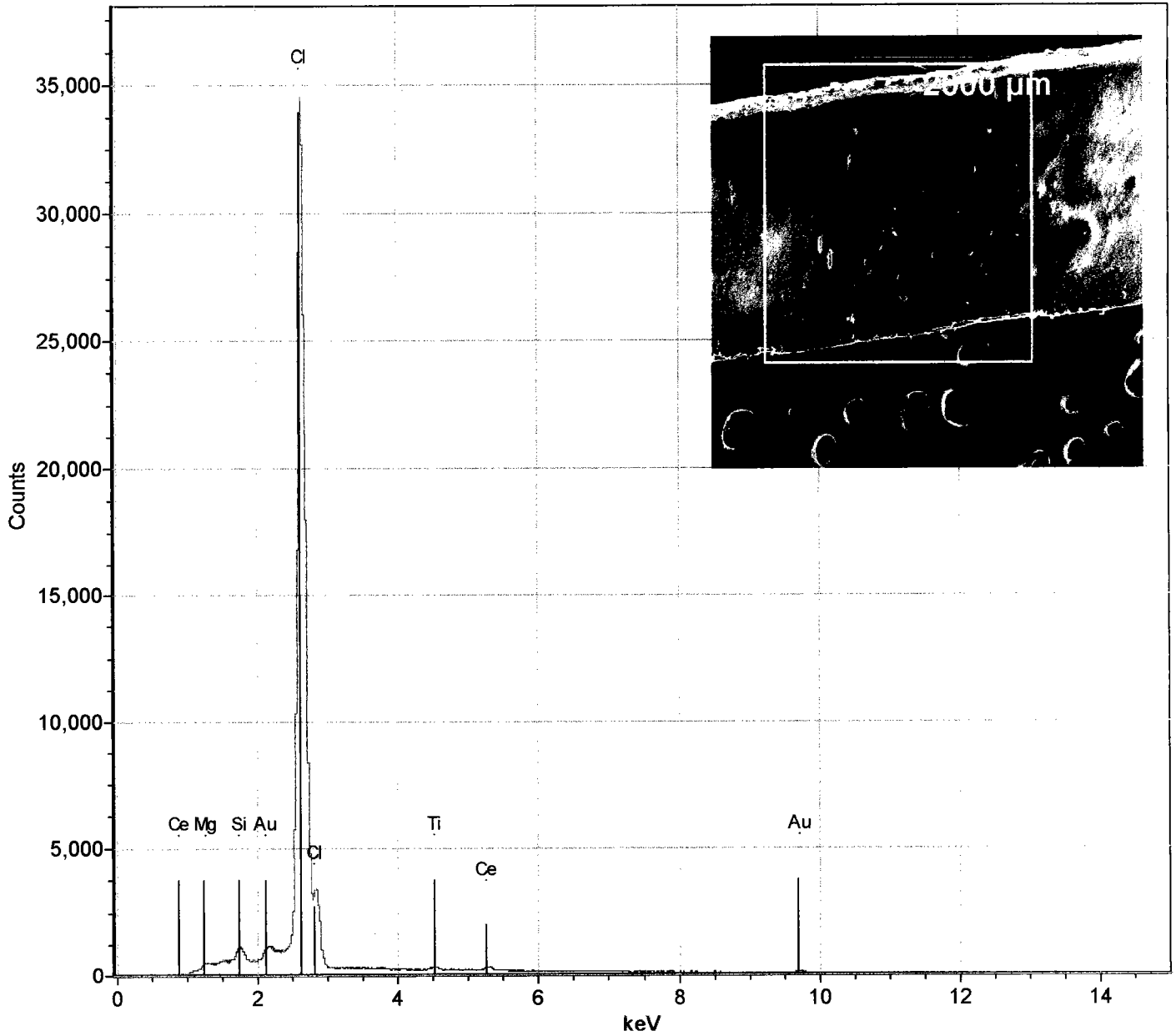
EDXA Elemental Profile using Aspex PSEM II SEM/EDXA
